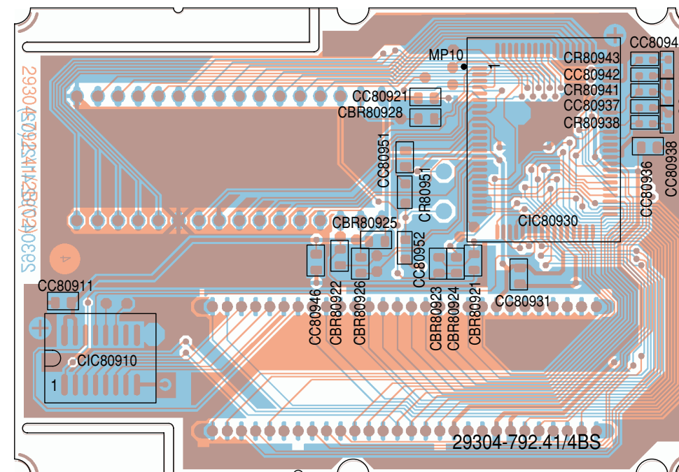
Bestückungsseite (SMD) / Component Side (SMD)
