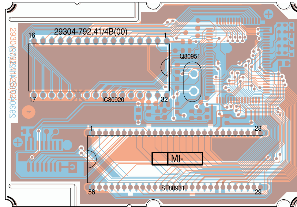
Bestückungsseite / Component Side
